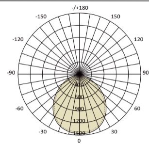
2X2 - 24W - RA80 - 4000K
